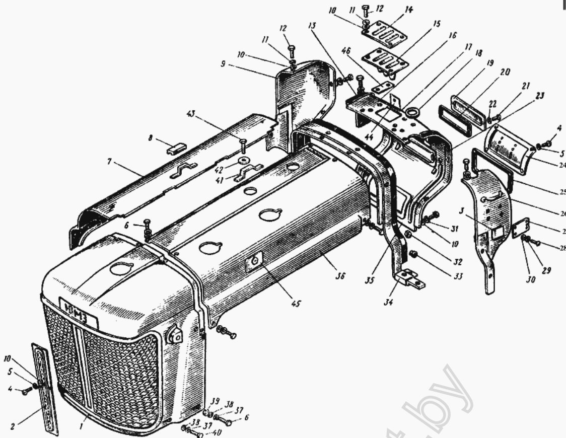
Рис. 74. Облицовка радиатора. Капот
